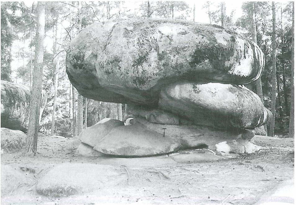
Abb. 4: „Pilzstein“ (524 m Seehöhe), Blockheide Gmünd-Eibenstein.
