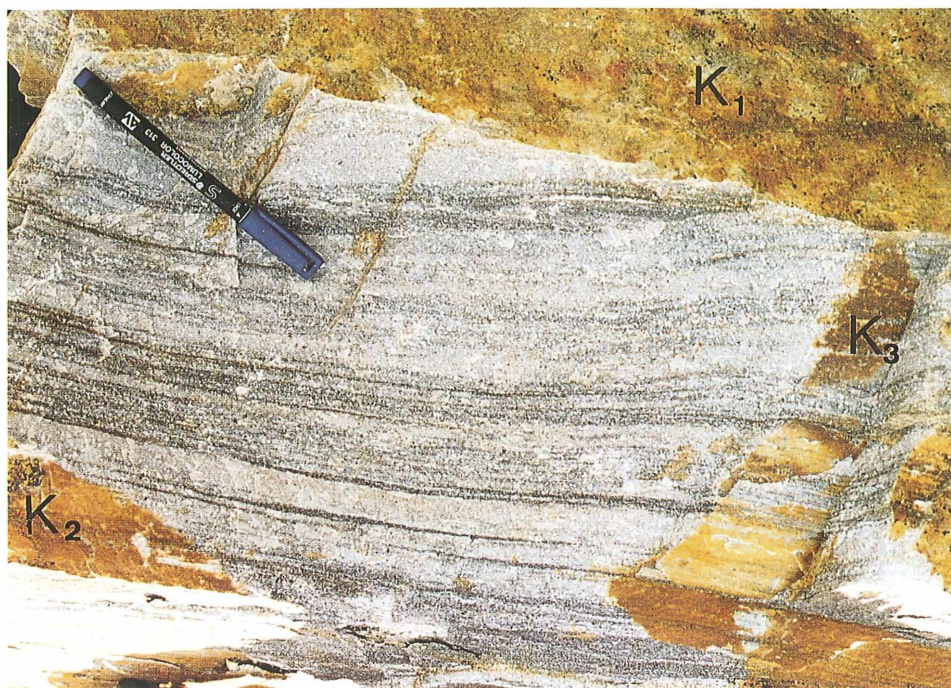
Abb. 3: Heller, feinkörniger und feingebänderter Granulit.
