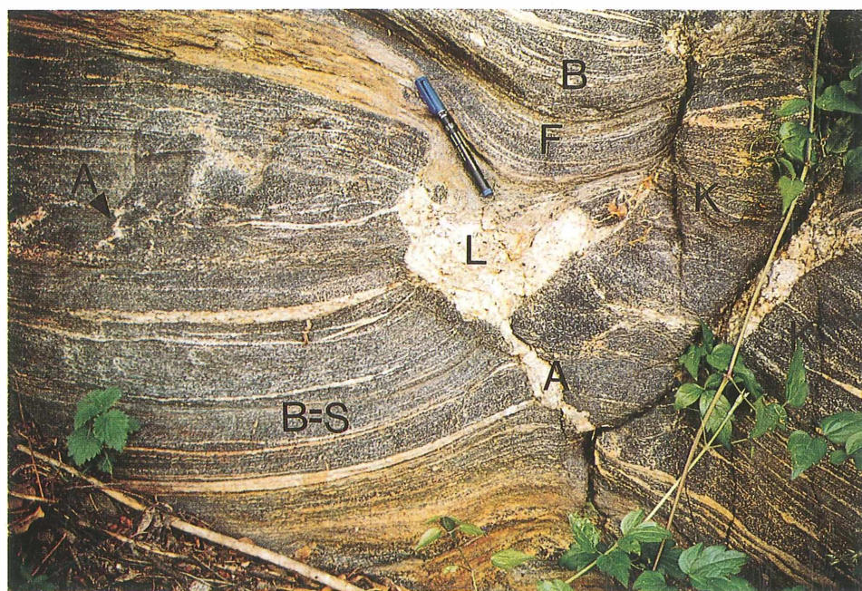
Abb 7: Migmatischer Amphibolit.
