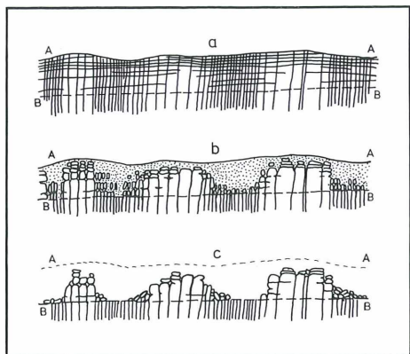
Abb. 6: Abhängigkeit der Felsburgbildung von der Kluftdichte (nach LINTON 1955, Fig. 2a-c).
