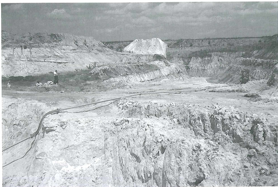
Abb. 2: Tongrube Fa. Frings bei Maiersch im Horner Becken, NÖ
