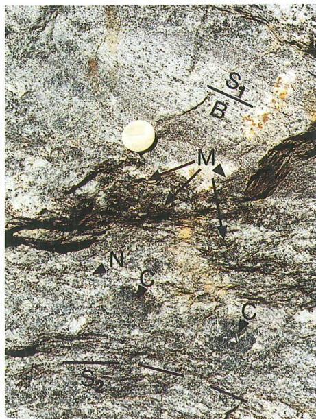
Abb. 9: Migmatischer Cordieritgneis der Monotonen Serie.
