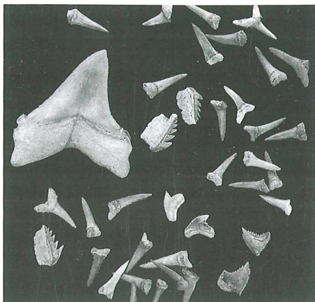
Abb. 4: Verschiedene Hai-Zähne (Untermiozän: Eggenburgium).
