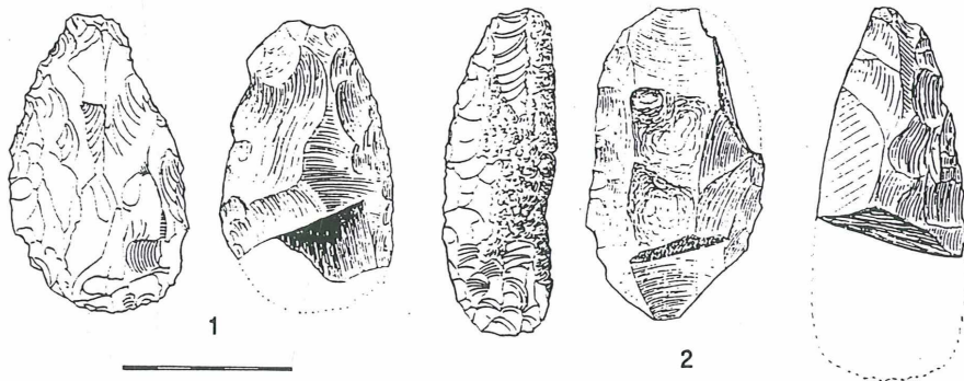
Abb. 3: Gudenushöhle im Kremstal.
