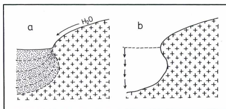
Abb. 15: Entstehung von Felsfuß-Hohlkehlen (modifiziert nach TWIDALE 1984, Fig. 9.13).
