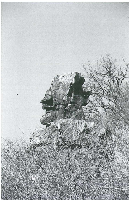
Granzer Jud (NÖ — ME — 005)
