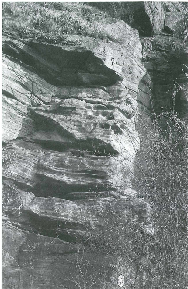
Kolke der Donau (NÖ — KR — 060)
