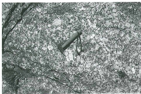
Abb. 2: Weinsberger Granit in Straßenaufschluß bei Langschlag.
