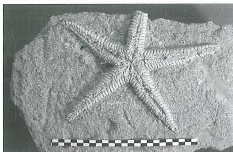
Abb. 8: Seestern ( Asteropecten sp.).
