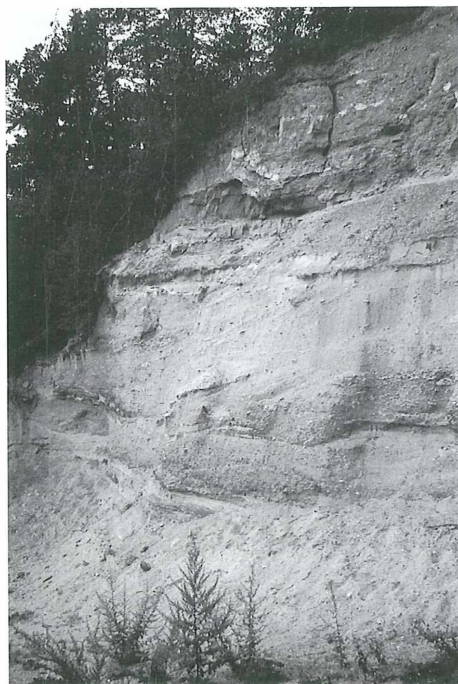
Abb. 3: Gemeindesandgrube bei Obernholz, Straßertal, NÖ
