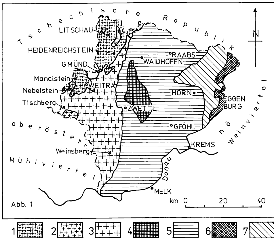
Abb. 1: Geologische Kartenskizze des kristallinen Grundgebirges des Waldviertels.
