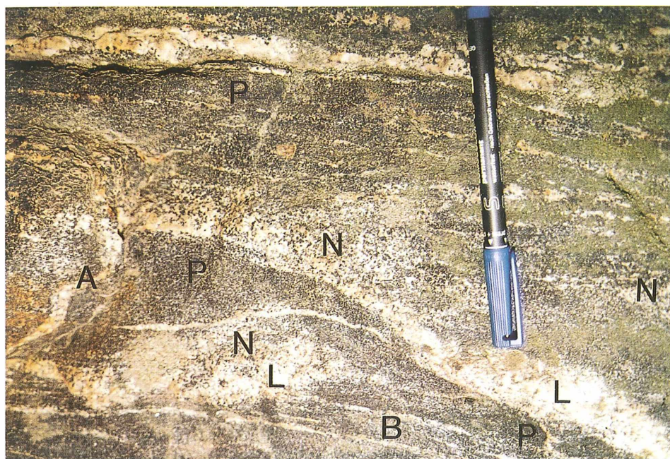
Abb. 8: Migmatischer Amphibolit.
